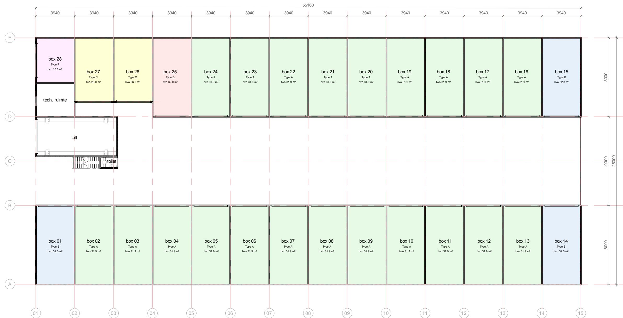
Plattegrond beganegrond 1 : 200
